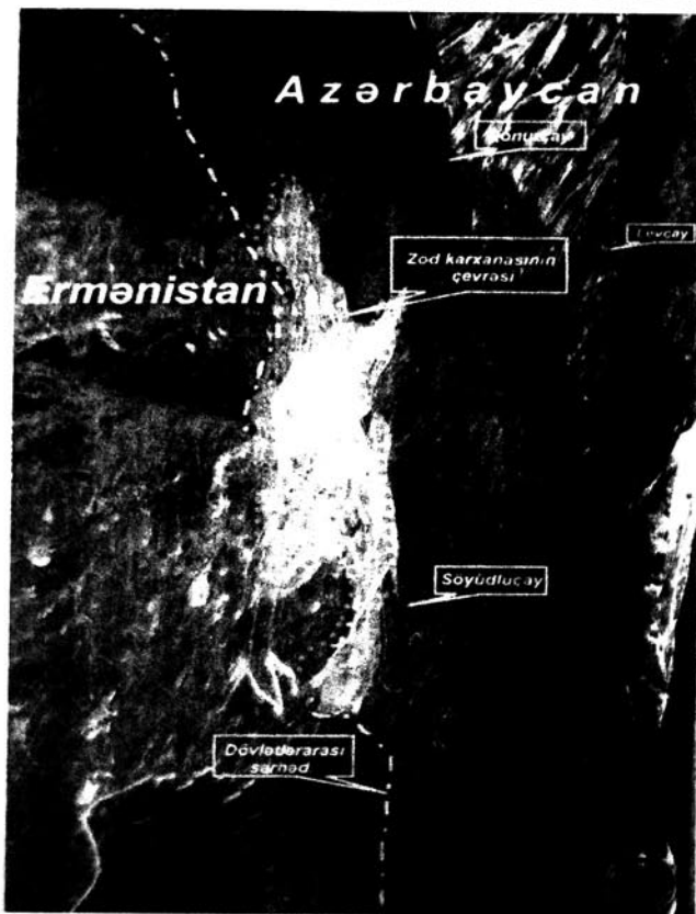
Şəkil 3. Soyüdlü (Zod) qızıl mədəni karxanasının peykdən görünüşü
